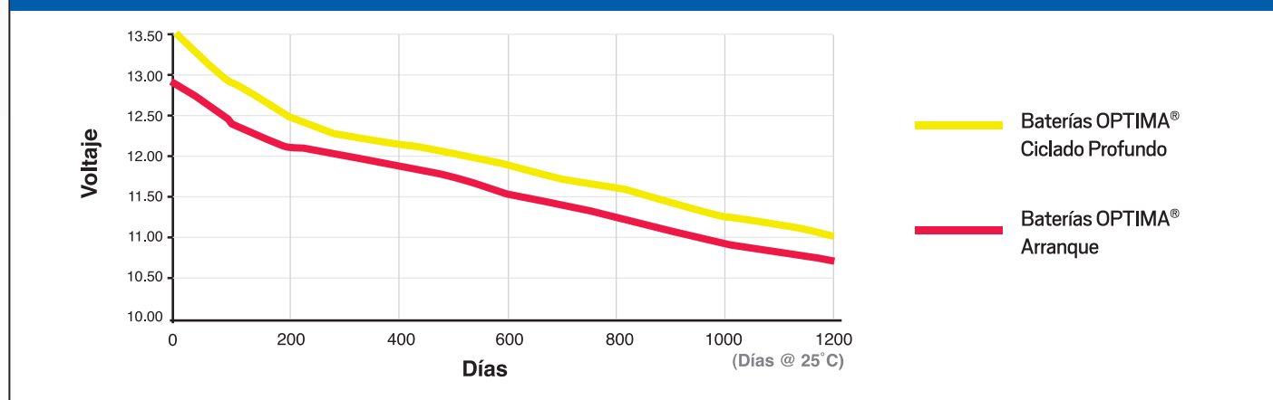
Voltaje Circuito Abierto vs Tiempo Anaque
